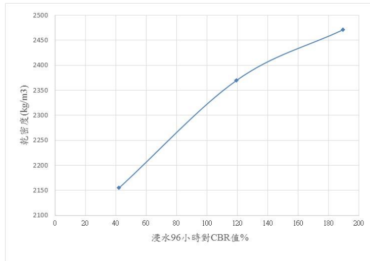
圖 3-1 A 氧化碴級配粒料乾密度與 CBR 關係圖 [23]
