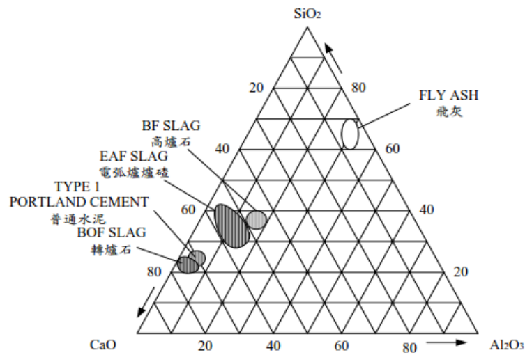
圖 2-4 氧化渣 \text{CaO-SiO}_2\text{-Al}_2\text{O}_3 三相圖 [16]
