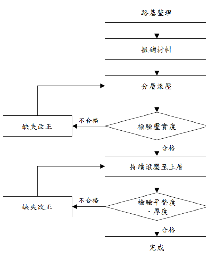
圖 5-1 道路級配粒料基底層施工流程
