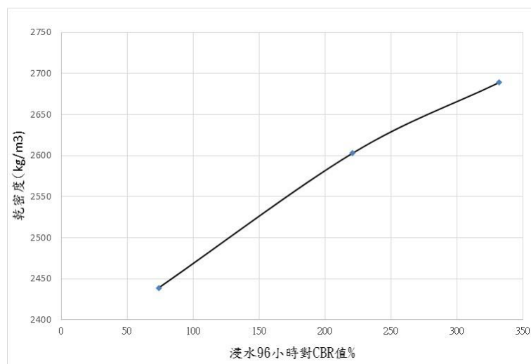
圖 3-2 B 氧化碴級配粒料乾密度與 CBR 關係圖 [24]
